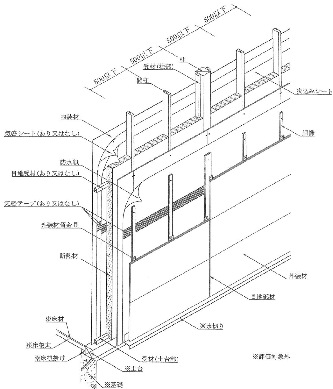
透視図 (銅縁仕様：構造用面材あり仕様)
