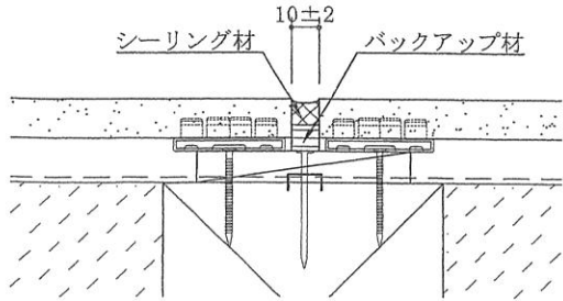
①シーリング材とバックアップ材の併用目地
