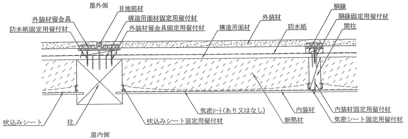
水平断面図 (胴縁仕様：構造用面材あり仕様)
