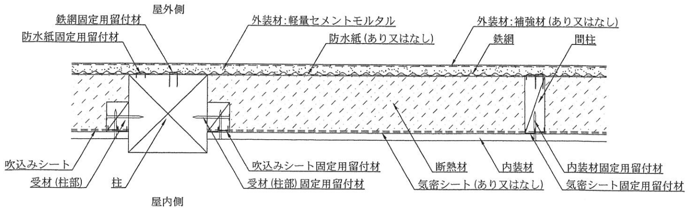
水平断面図(直張仕様) (構造用面材なし・下地材なし仕様)
