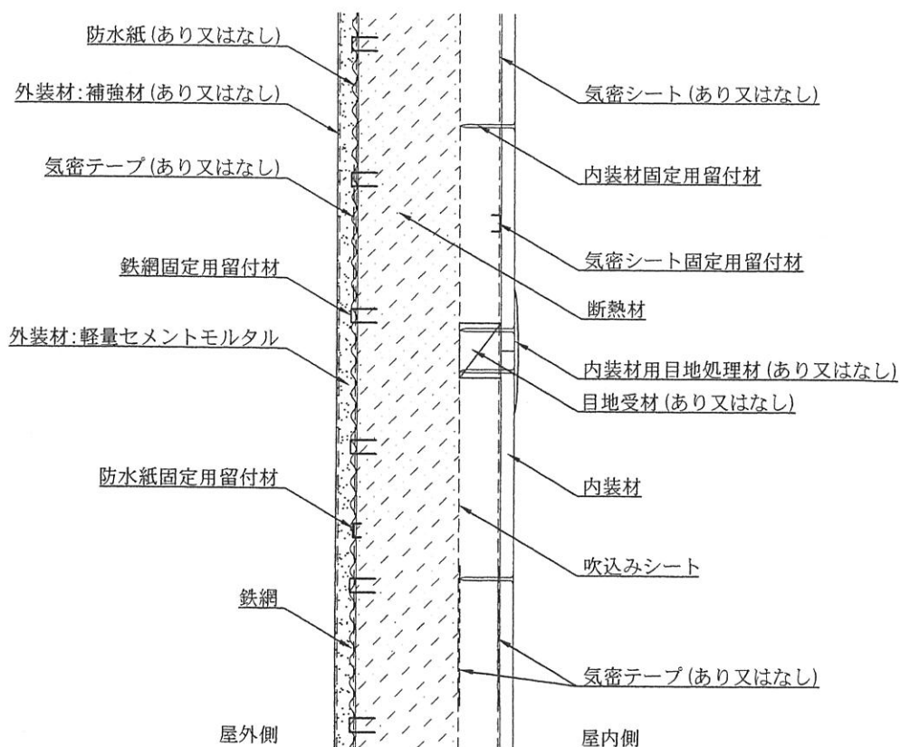
鉛直断面図 (直張仕様) (構造用面材なし・下地材なし仕様)
