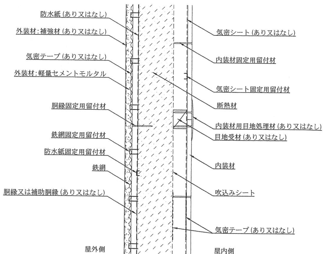
鉛直断面図 (通気仕様) (構造用面材なし・下地材なし仕様)
