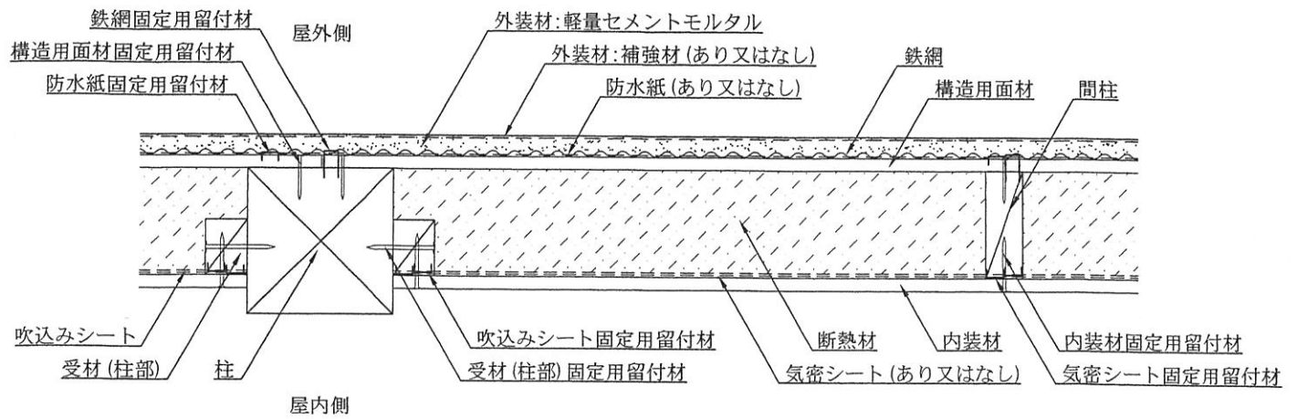
水平断面図 (直張仕様) (構造用面材あり・下地材なし仕様)
