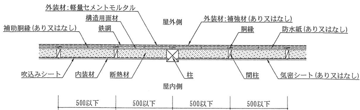
水平断面図 (通気仕様) (構造用面材あり・下地材なし仕様)
