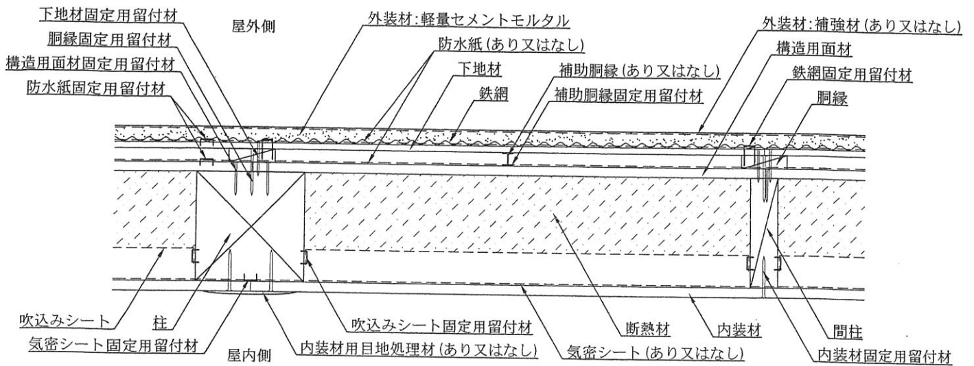
水平断面図 (通気仕様) (構造用面材あり・下地材あり仕様)
