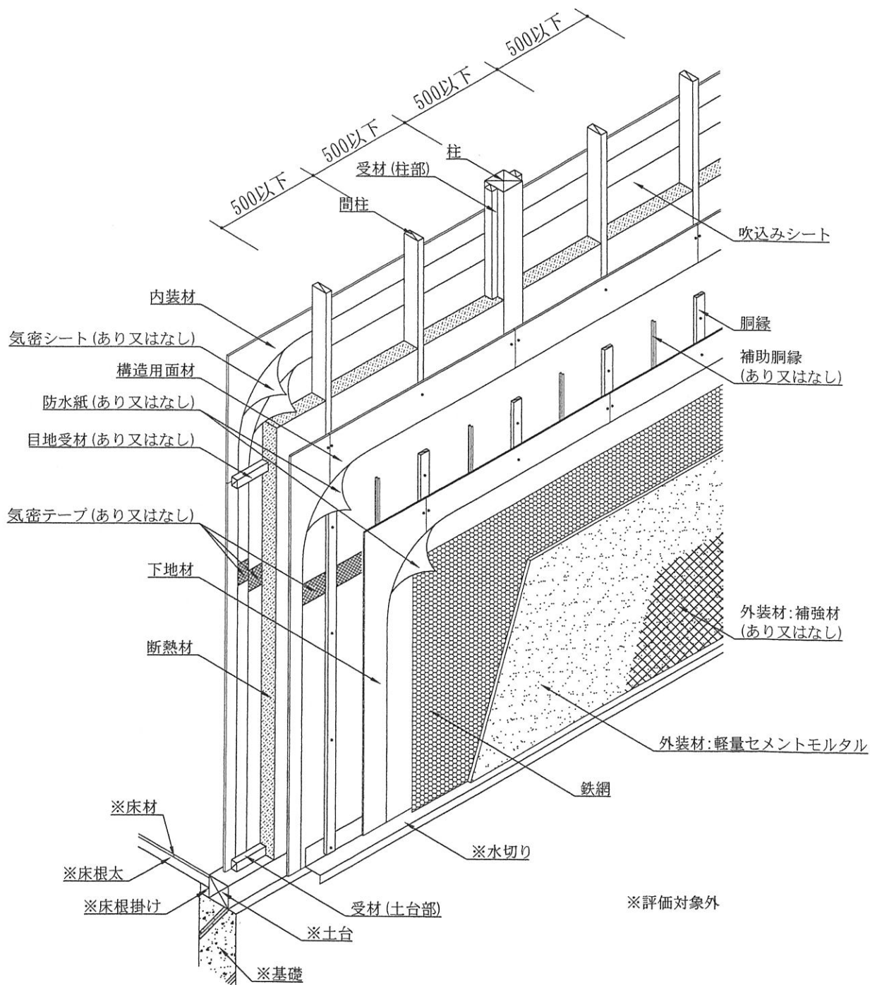
透視図(通気仕様) (構造用面材あり・下地材あり仕様)
