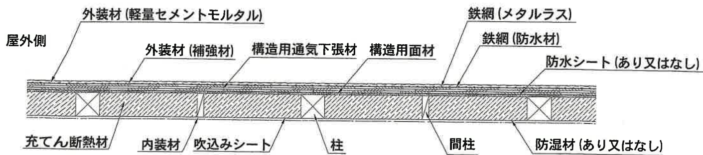
水平断面図
