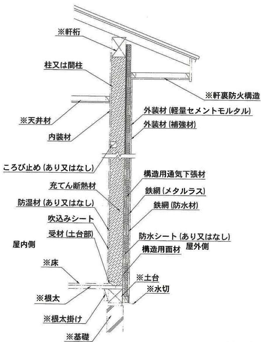
鉛直断面図
