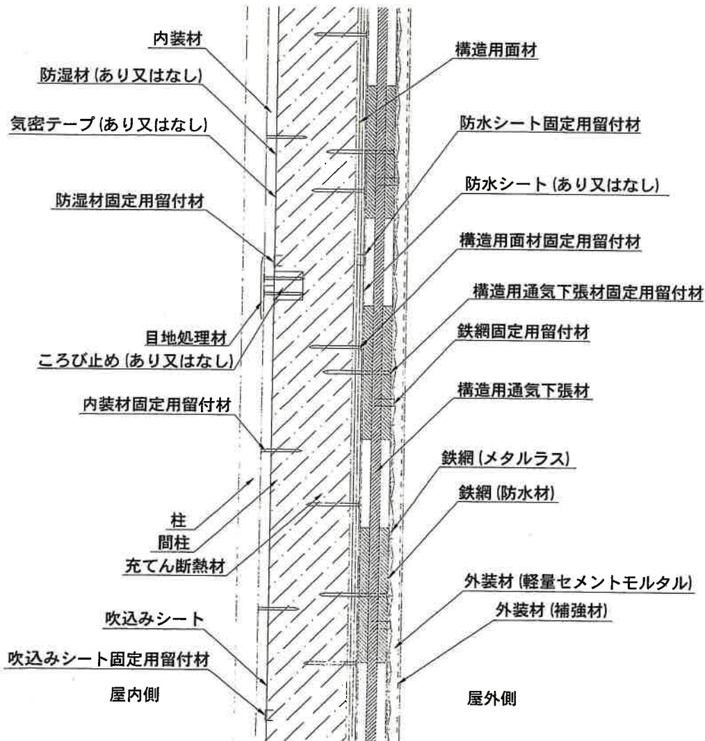
鉛直断面図
