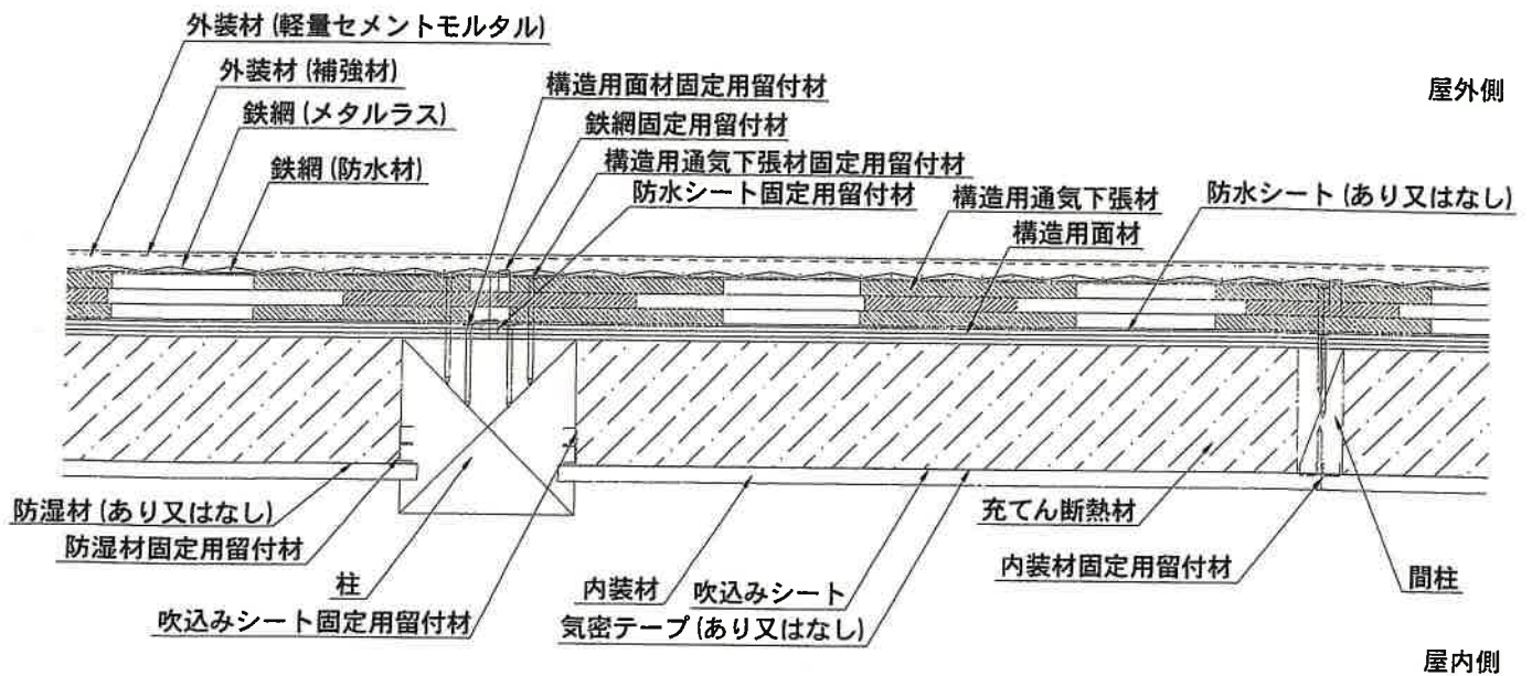
水平断面図
