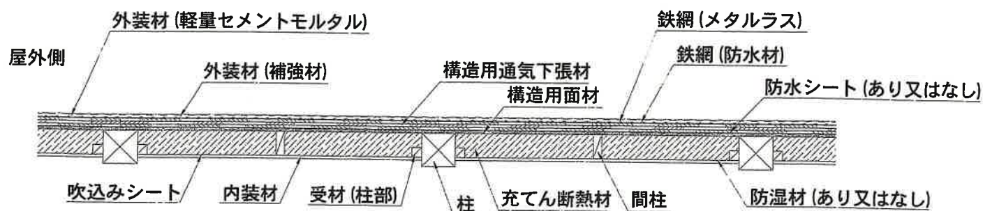
水平断面図
