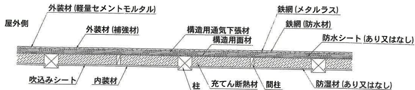
水平断面図
