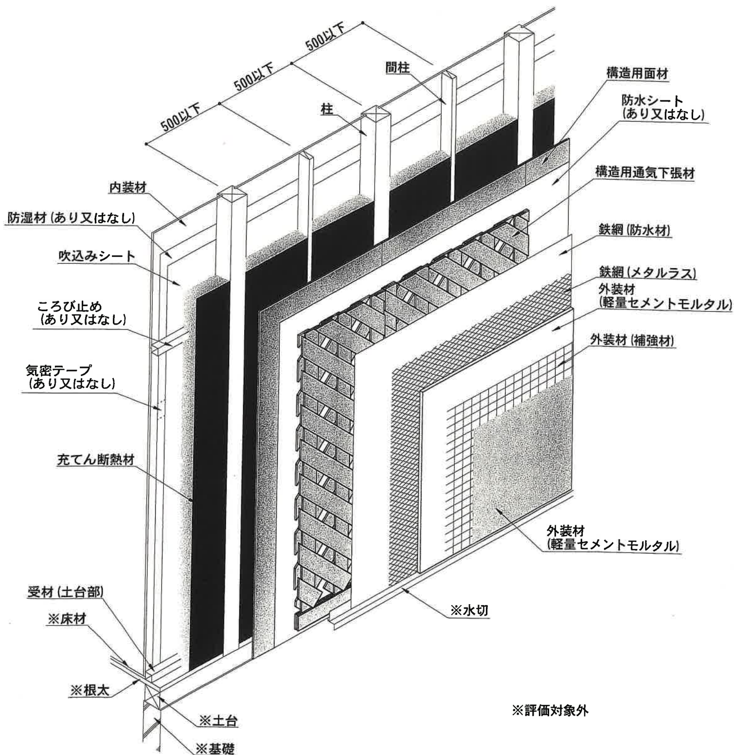
透視図 (欠き込み真壁造：構造用面材あり仕様)
