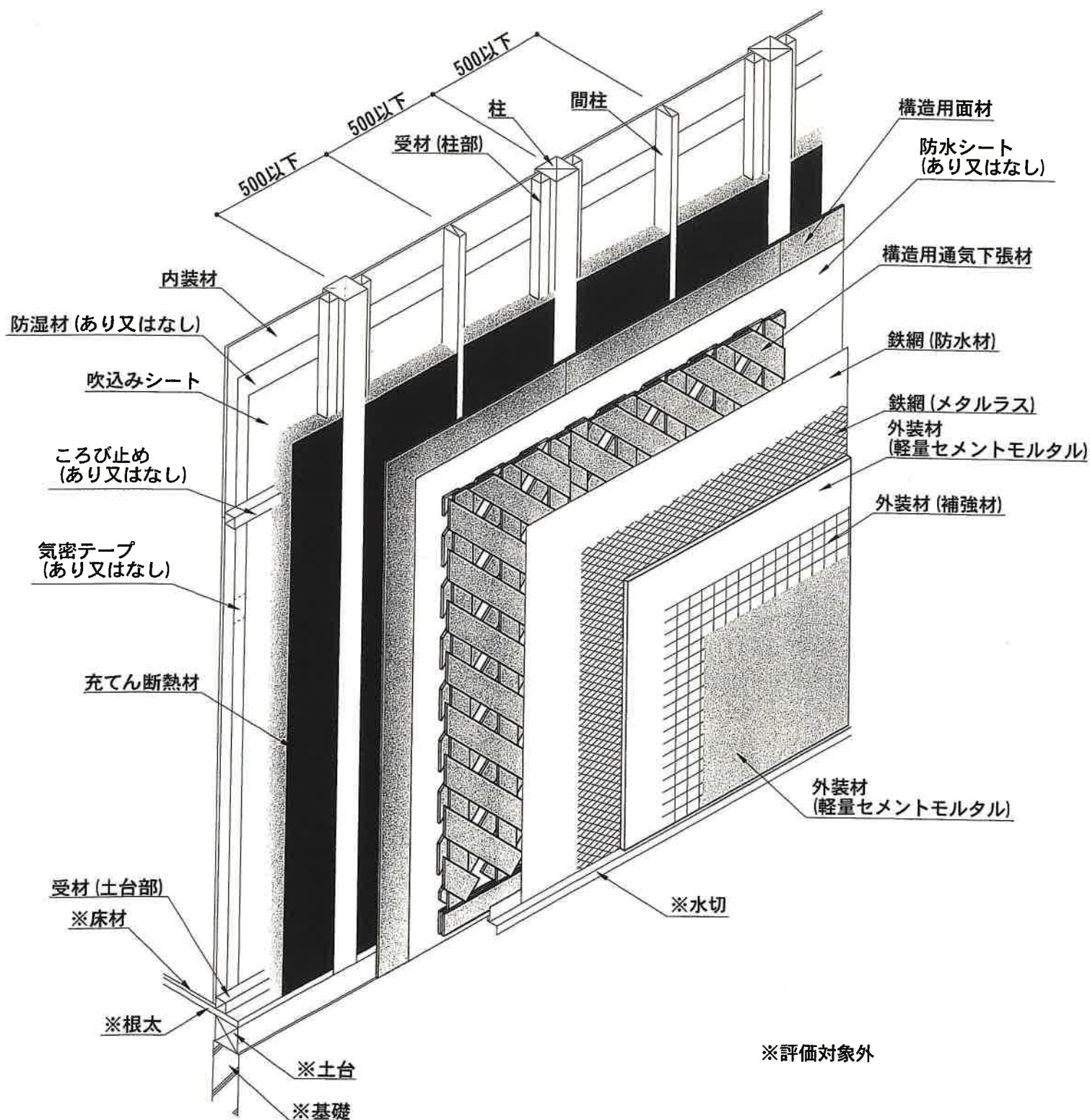
透視図 (受材真壁造：構造用面材あり仕様)
