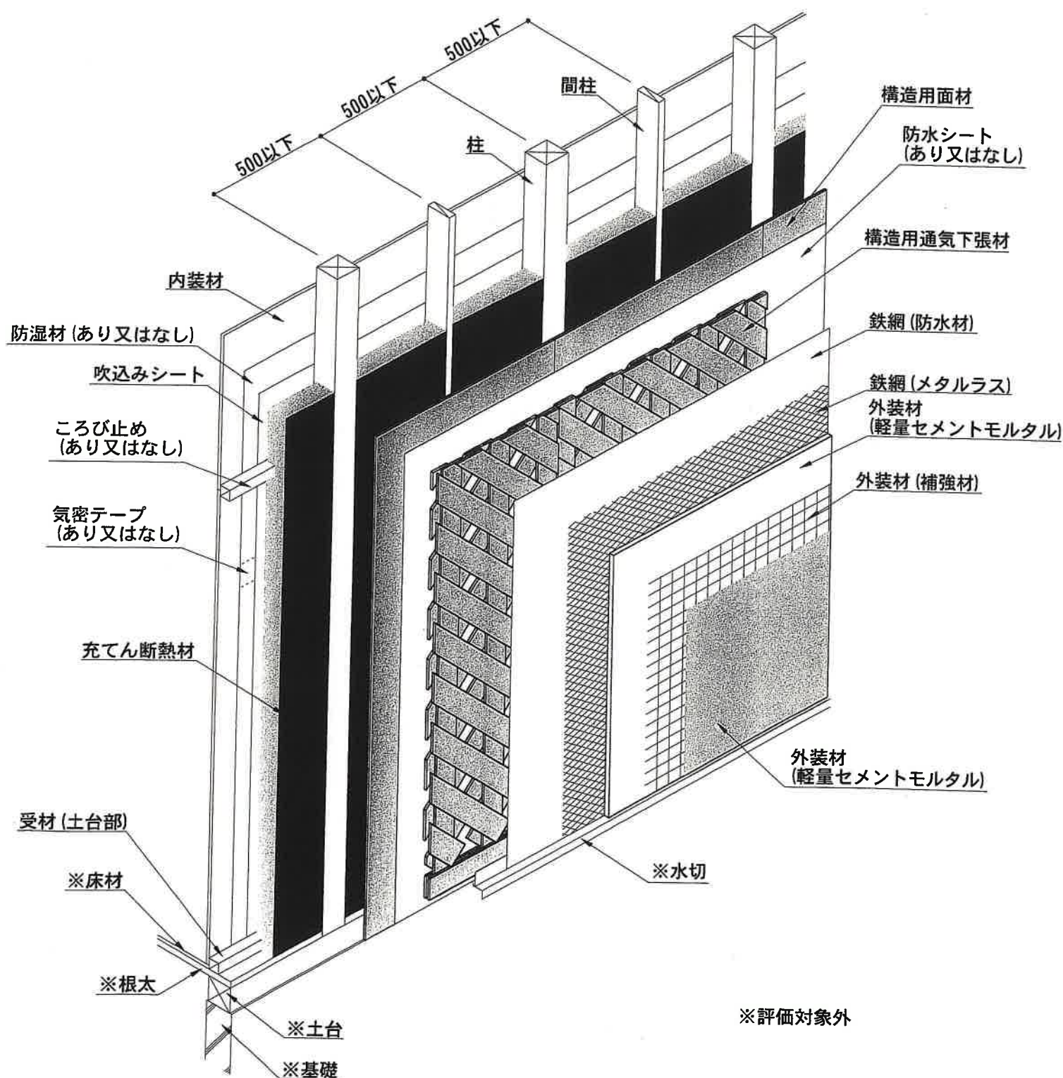
透視図(大壁造:構造用面材あり仕様)
