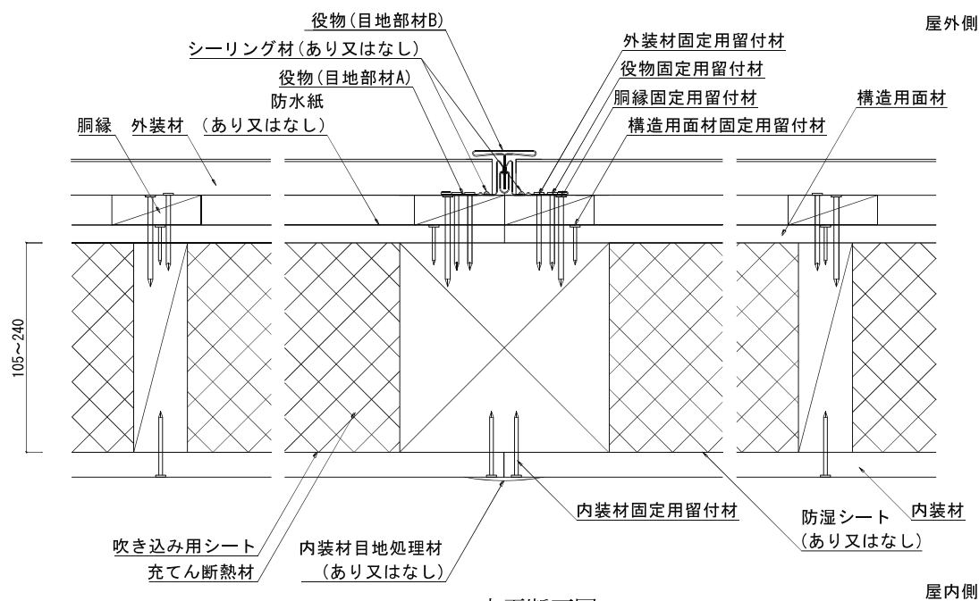
水平断面図
