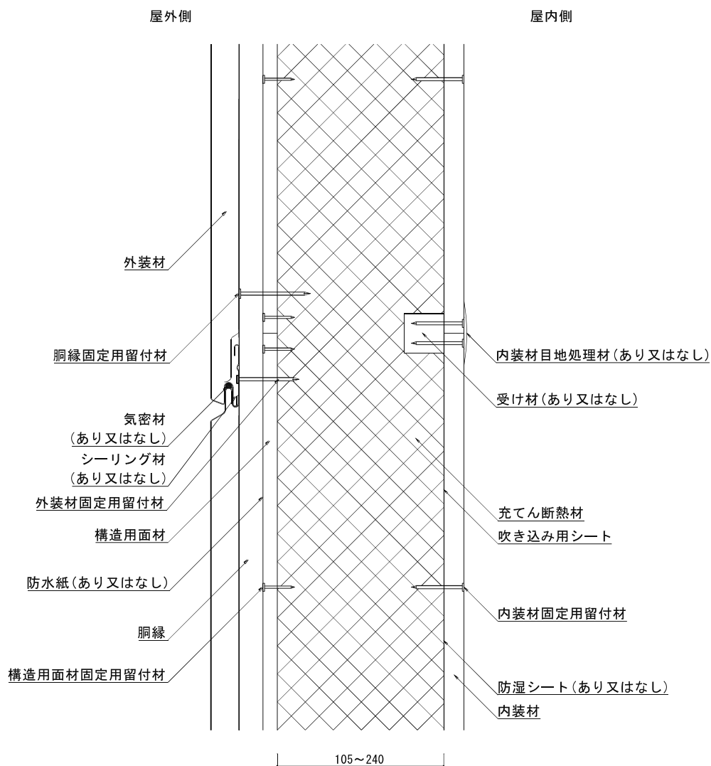
鉛直断面図
