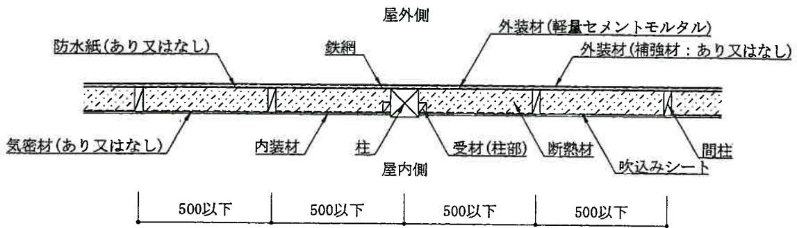
水平断面図 (受材真壁造・直張仕様)
