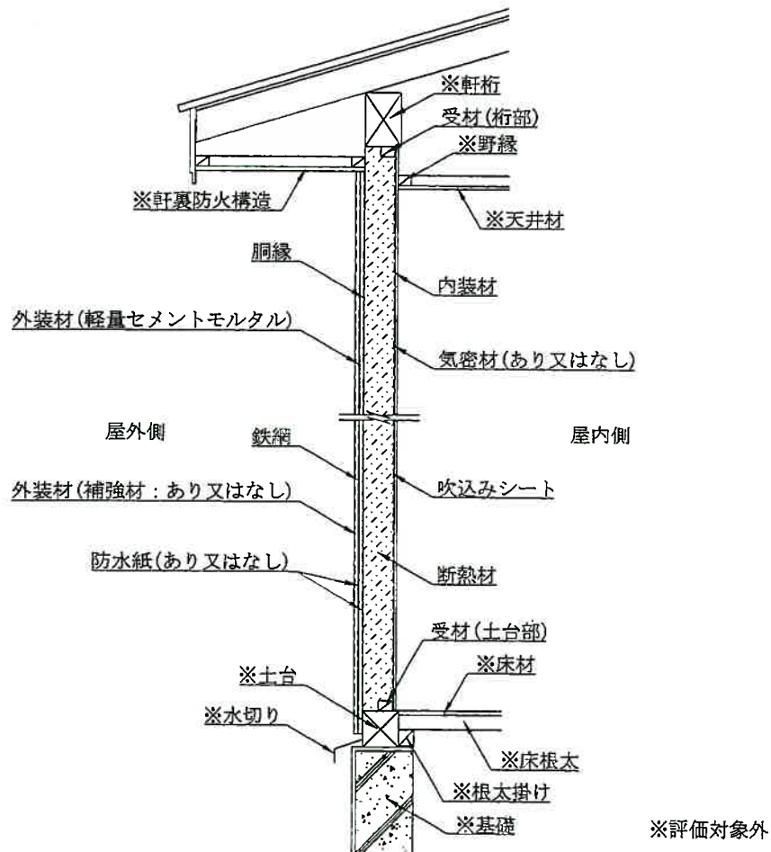
鉛直断面図 (受材真壁造・窓縁仕様)
