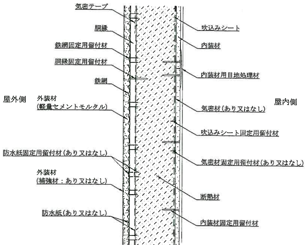
鉛直断面図 (欠き込み真壁造・胴縁仕様)
