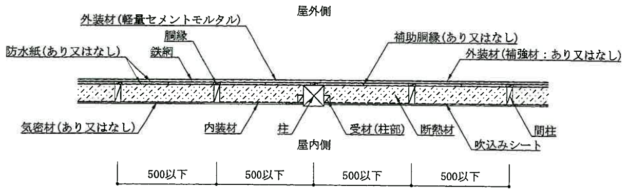
水平断面図 (受材真壁造・窓縁仕様)
