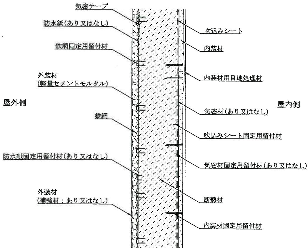
鉛直断面図 (欠き込み真壁造・直張仕様)
