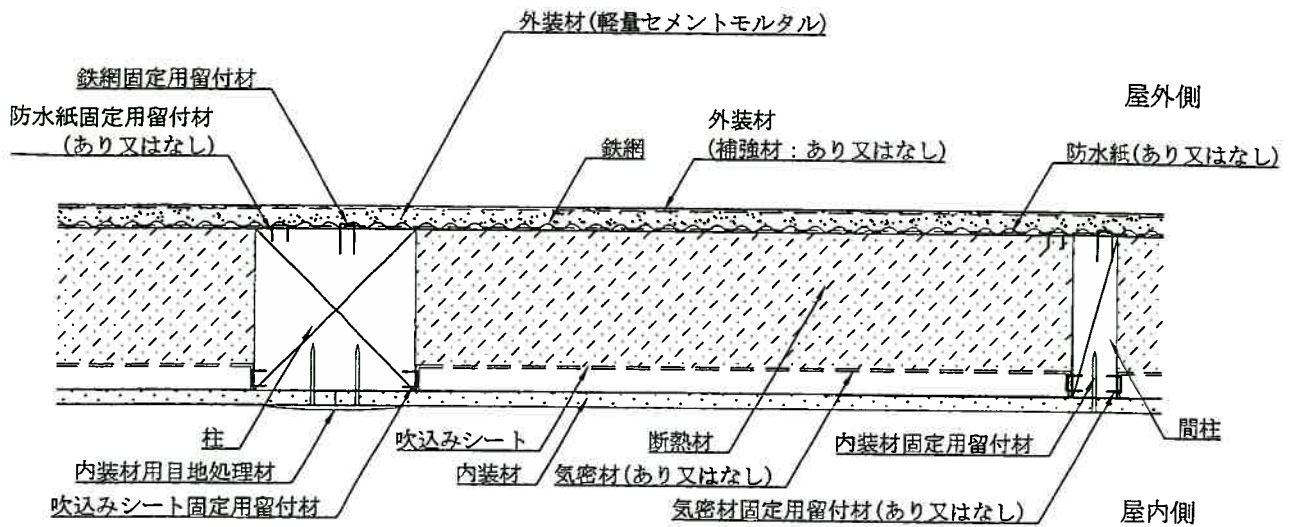
水平断面図 (大壁造・直張仕様)
