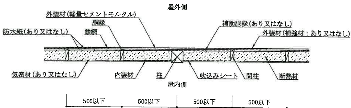
水平断面図 (欠き込み真壁造・胴縁仕様)
