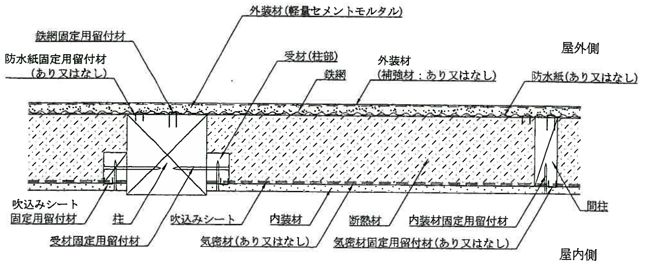
水平断面図 (受材真壁造・直張仕様)
