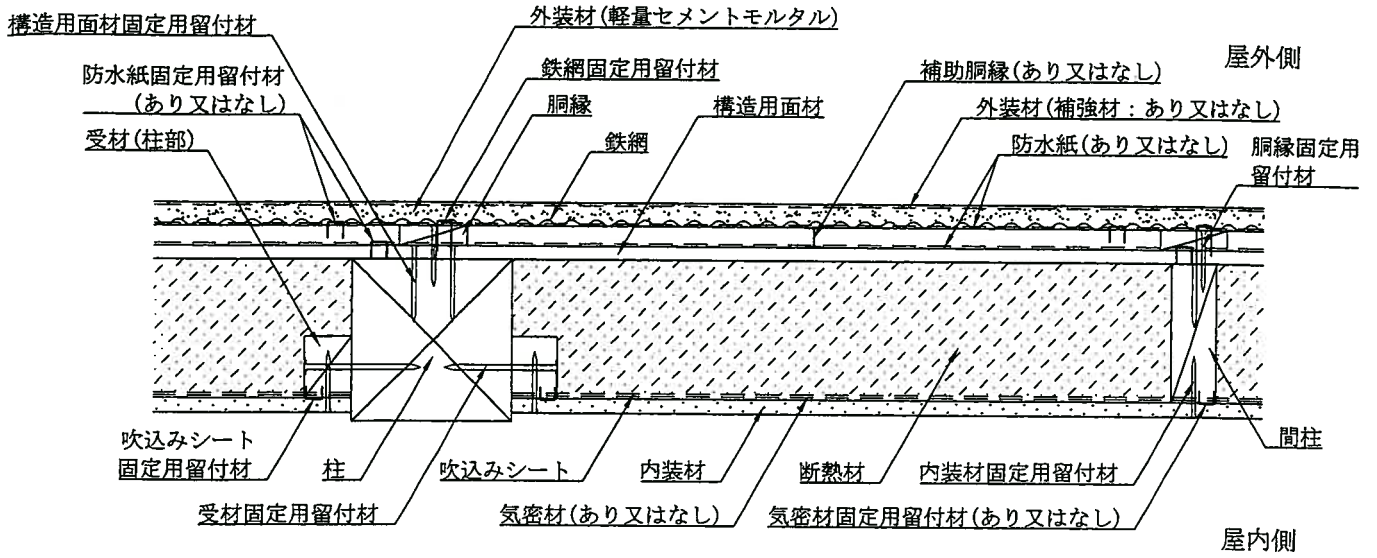
水平断面図 (受材真壁造・胴縁仕様)
