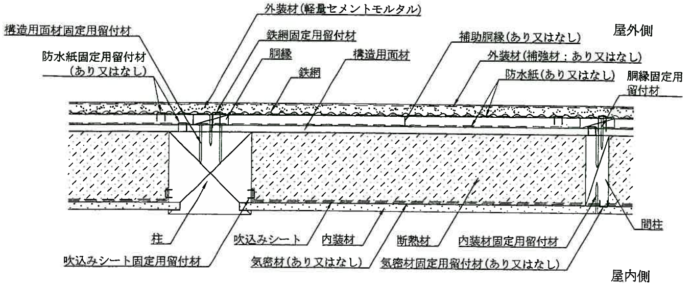
水平断面図 (欠き込み真壁造・胴縁仕様)
