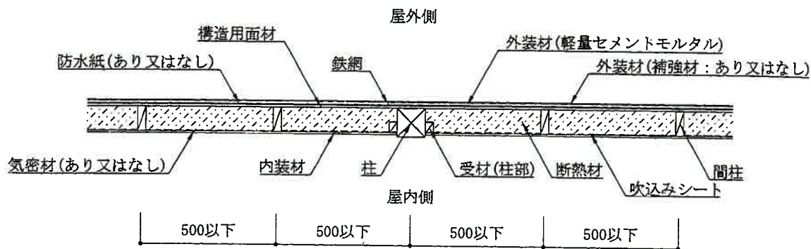
水平断面図 (受材真壁造・直張仕様)
