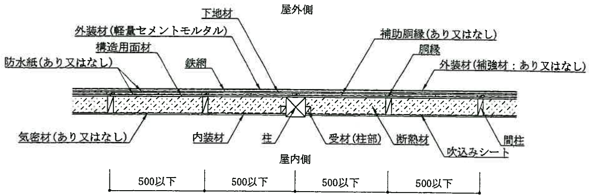
水平断面図 (受材真壁造・胴縁仕様)
