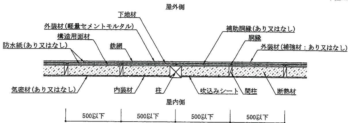
水平断面図 (欠き込み真壁造・胴縁仕様)
