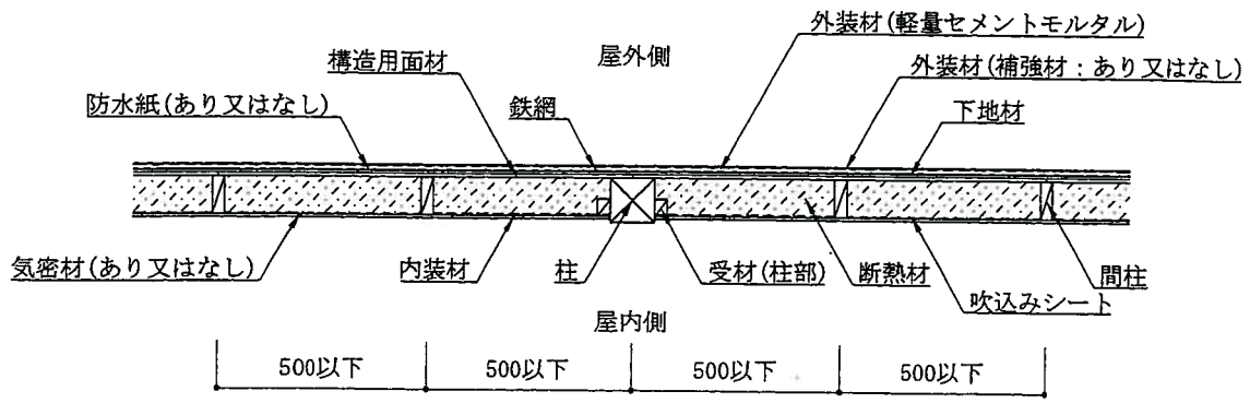
水平断面図 (受材真壁造・直張仕様)
