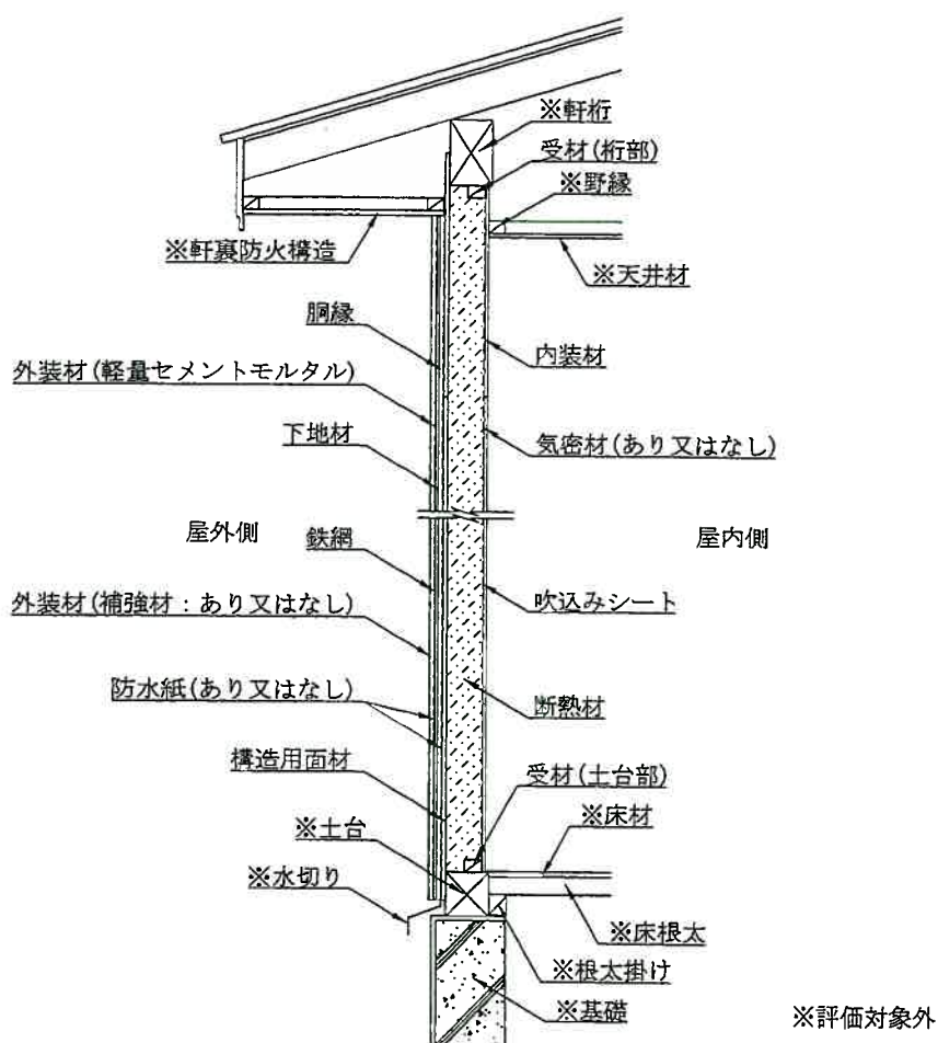
鉛直断面図 (受材真壁造・胴縁仕様)
